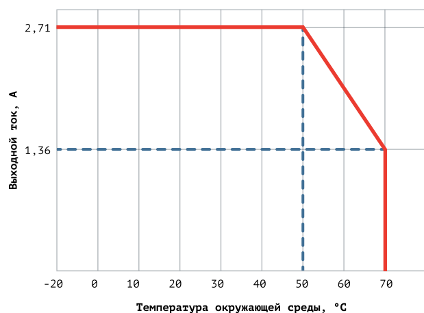
График снижения мощности в зависимости от температуры окружающей среды.
